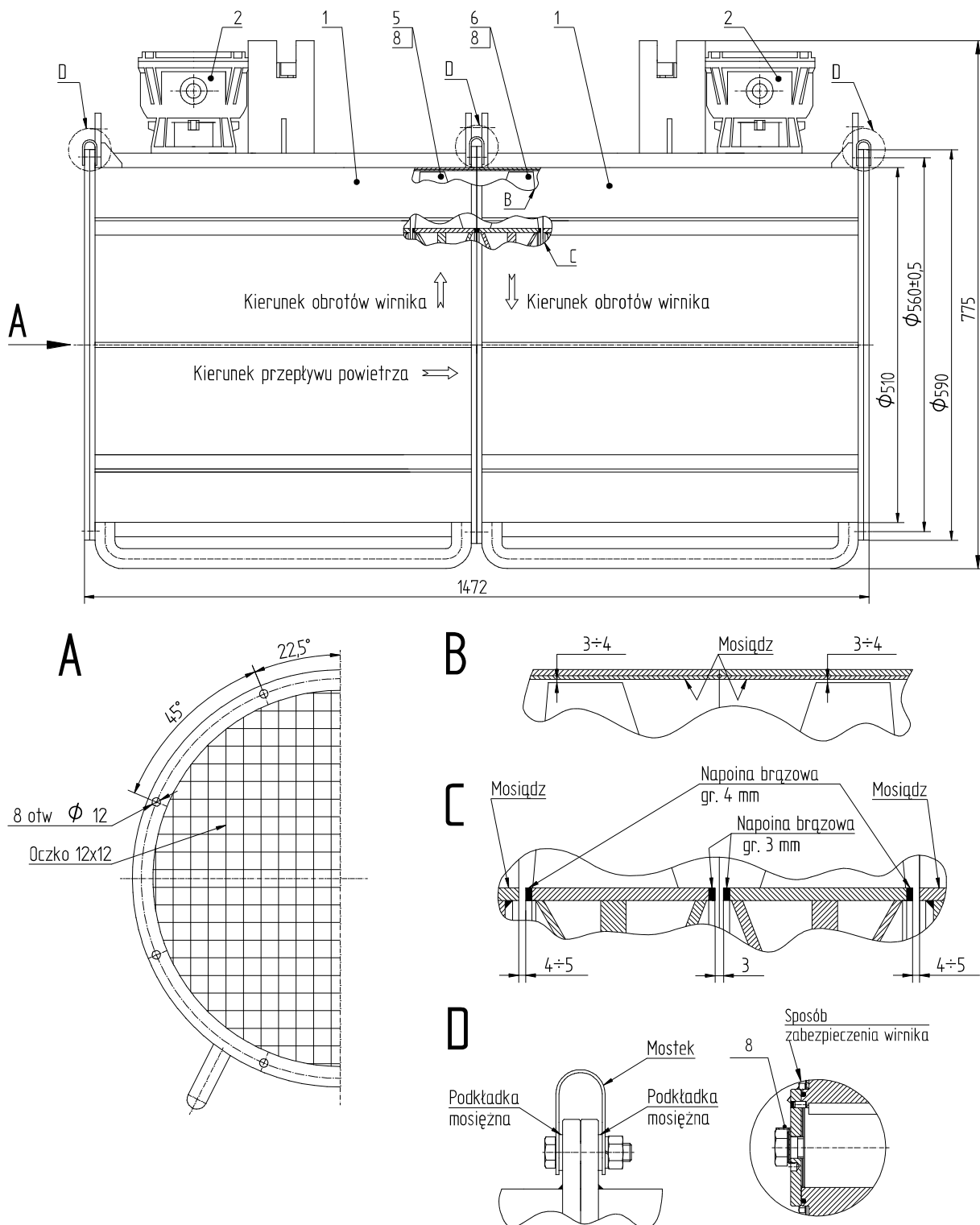
Rysunek 2 Wymiary gabarytowe wentylatora WLE-505A/SK
